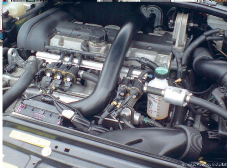
Instalacja piątej generacji z bezpośrednim wtryskiem gazu ciekłego
